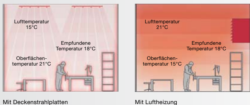
Abb.1: Lufttemperatur und Empfindungstemperatur
