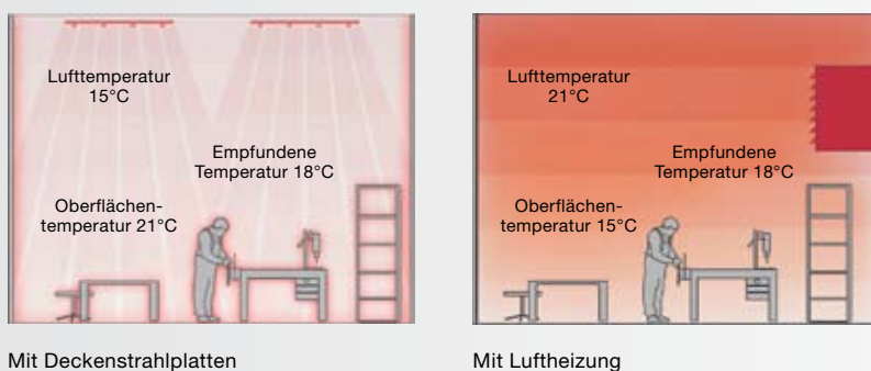
Abb.1: Lufttemperatur und Empfindungstemperatur
