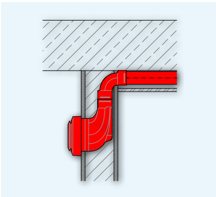
Zuluftdurchlass Wand und Lüftungsrrohr in der Decke
